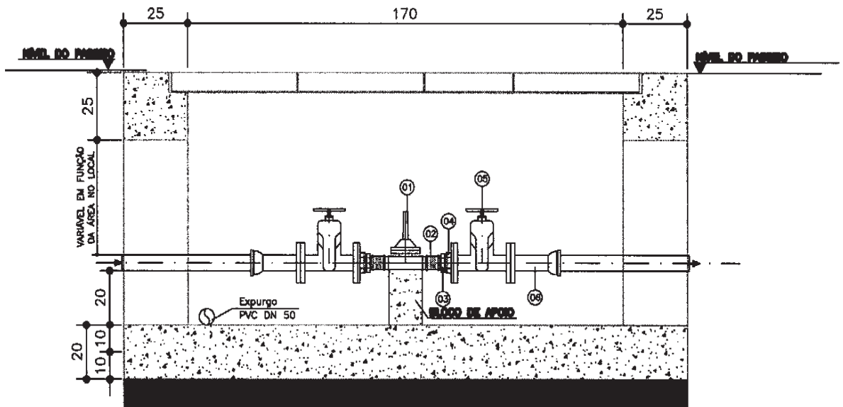
CORTE AA
